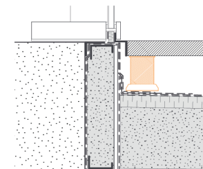
Dallage sur plots
